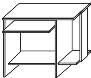
Ск-05 900x550x760
