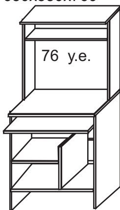
Ск-03н 650x550x1470
